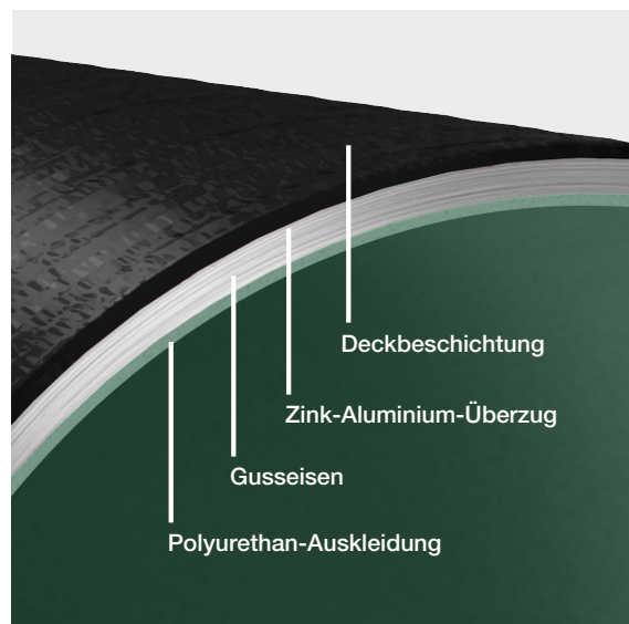
Wasserversorgung
